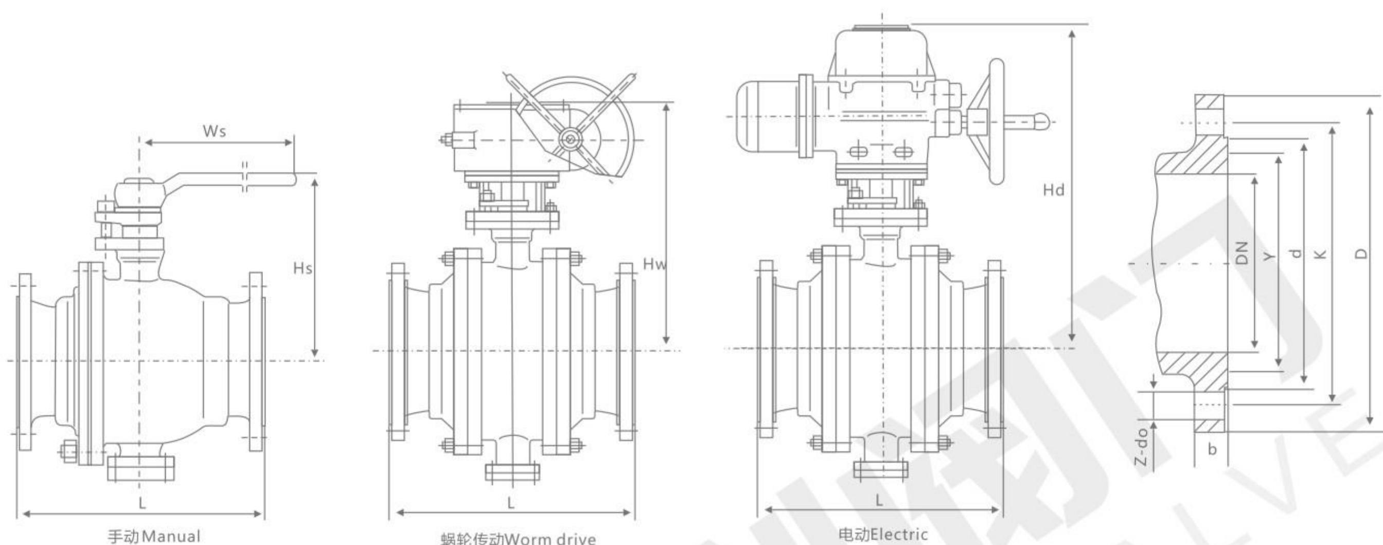
主要连接尺寸 Main connection dimensions
