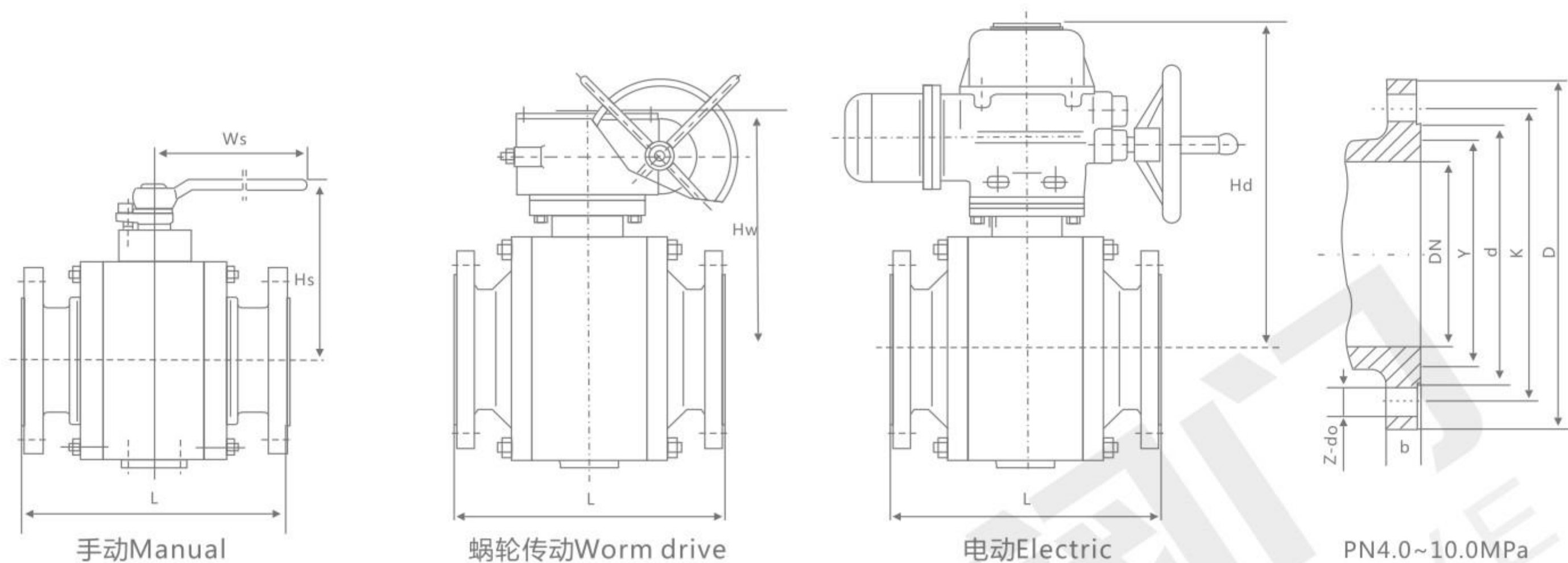
主要连接尺寸 Main connection dimensions
