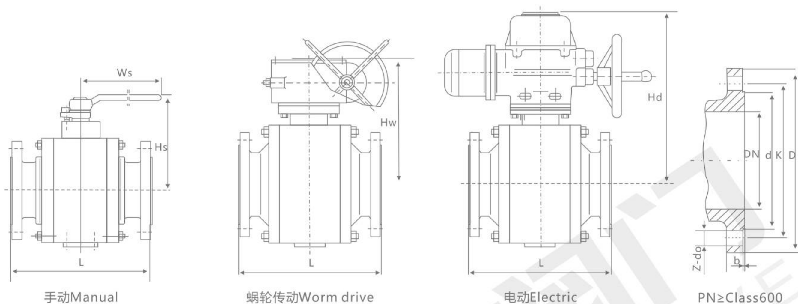
主要连接尺寸 Main connection dimensions
