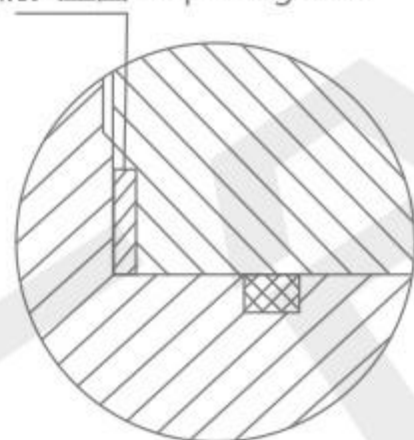
中法兰防火结构 Middle flange fireproof structure
