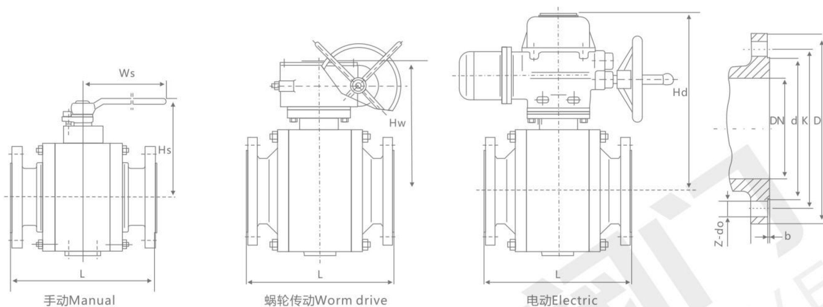
主要连接尺寸 Main connection dimensions
