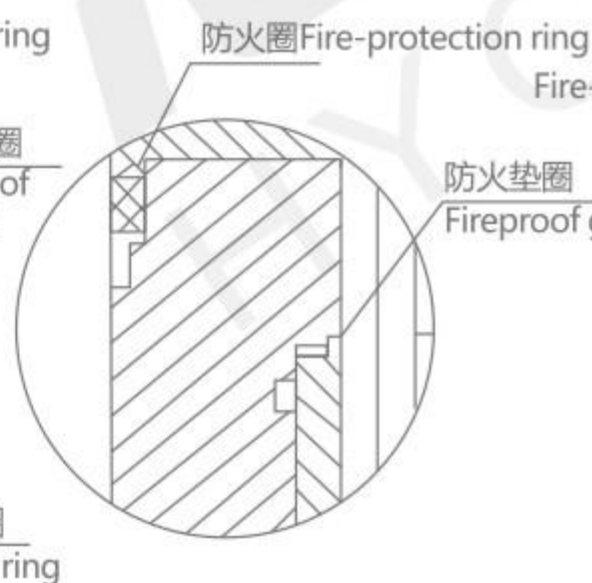
中法兰防火结构 Middle flange fireproof structure
