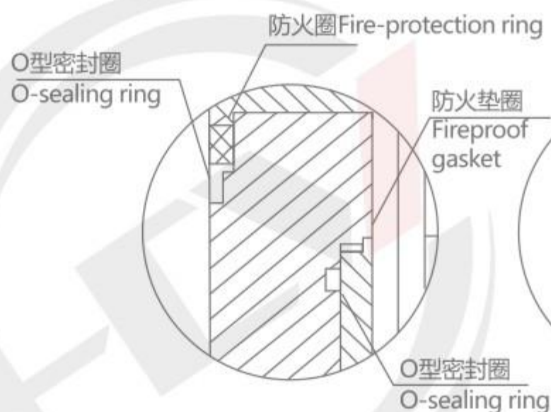
中法兰防火结构 Middle flange fireproof structure
