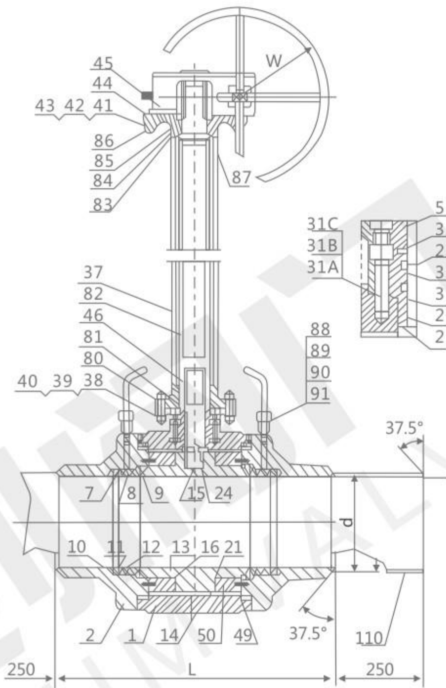
结构图Structure diagram
